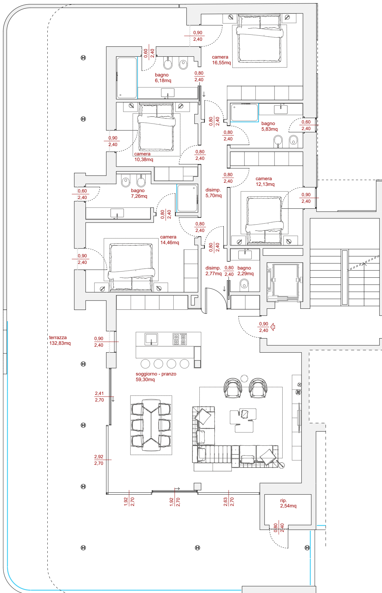
PIANTA PIANO SESTO
